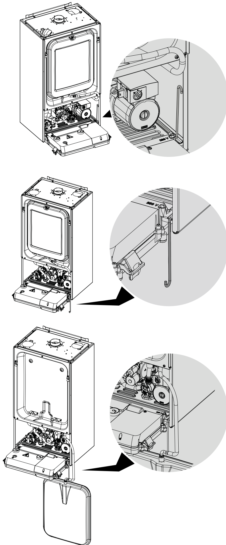
Рис. 37 Скоба для закрепления расширительного бака
