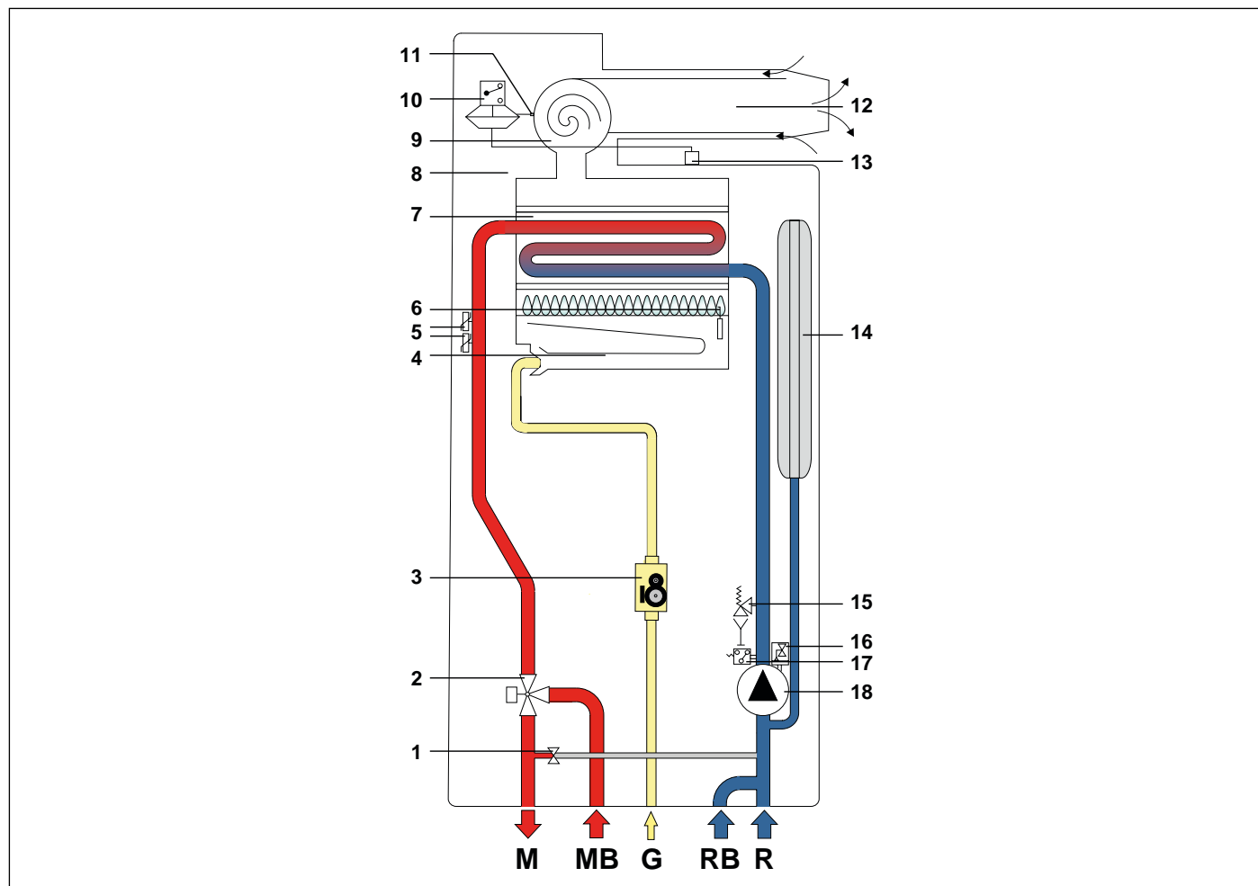
Рис. 7 Гидравлические схемы RBTFS
