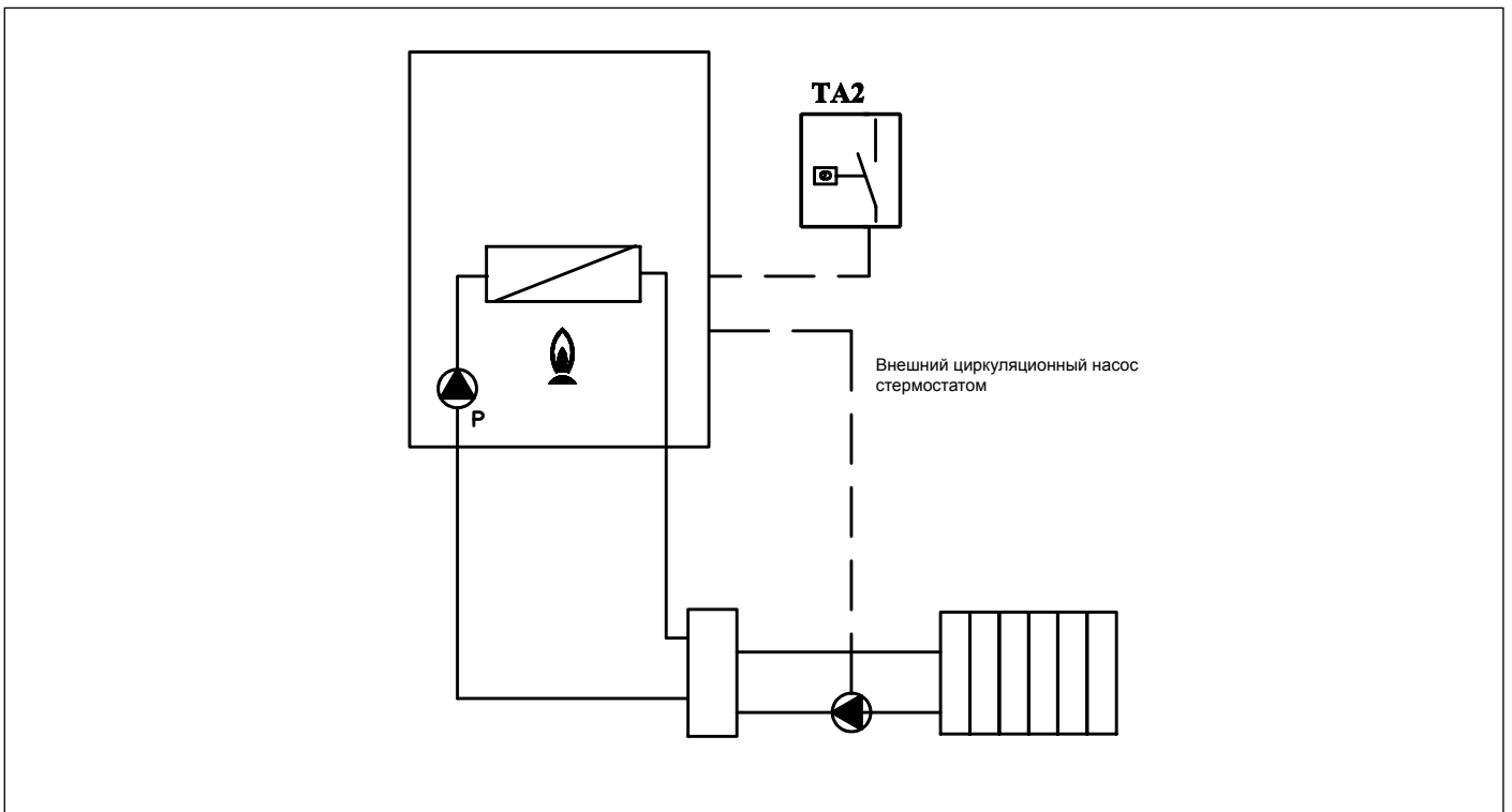
Рис. 33 Работа реле по внешнему запросу (P17=3)
