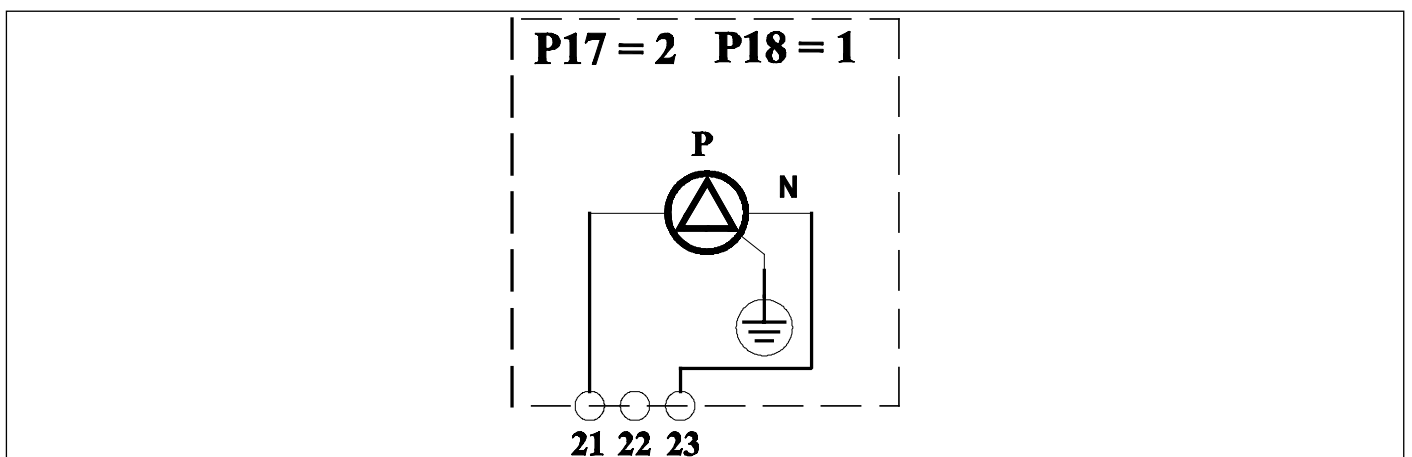
Рис. 27 Схема подключения multifunctional реле
