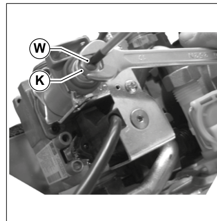
Рис. 41 Регулировка газового клапана
