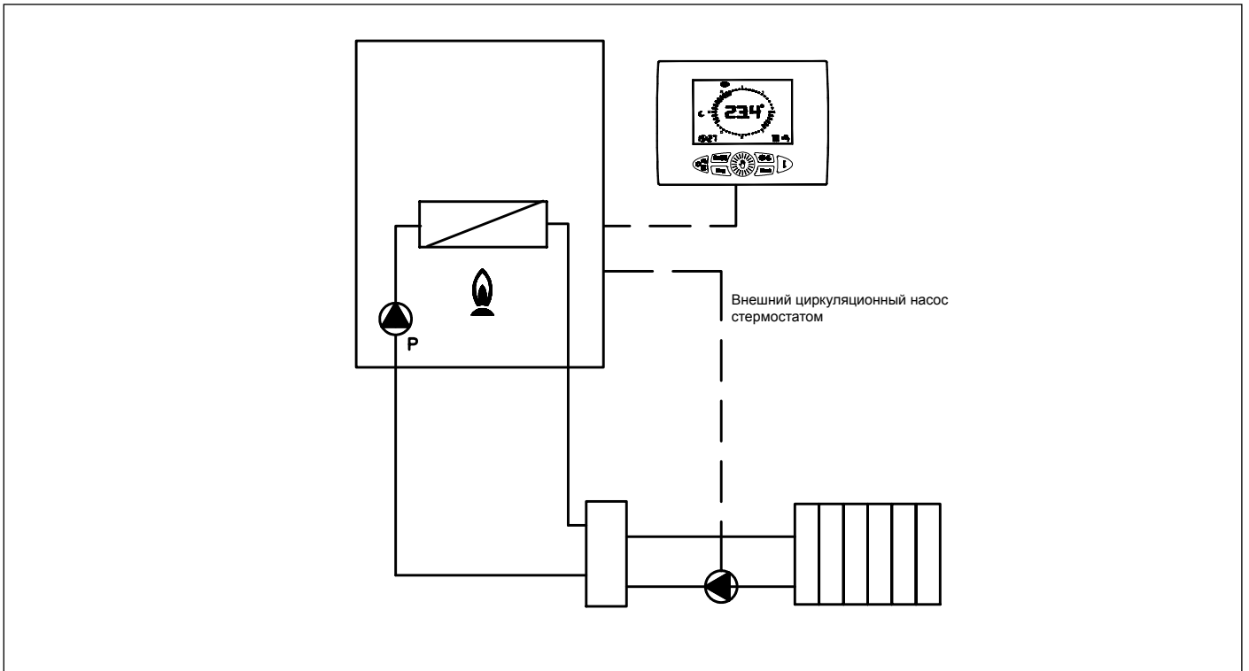
Рис. 32 Работа реле по внешнему запросу (P17=1)
