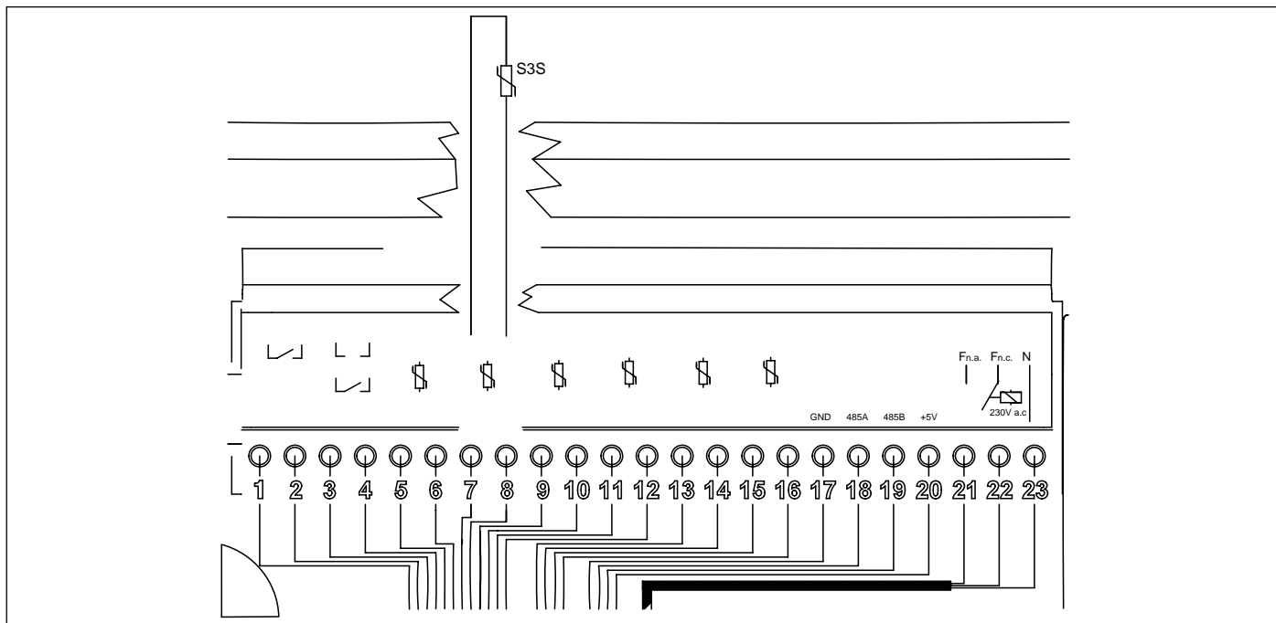
Рис. 25 Подробная электрическая схема CTFS
